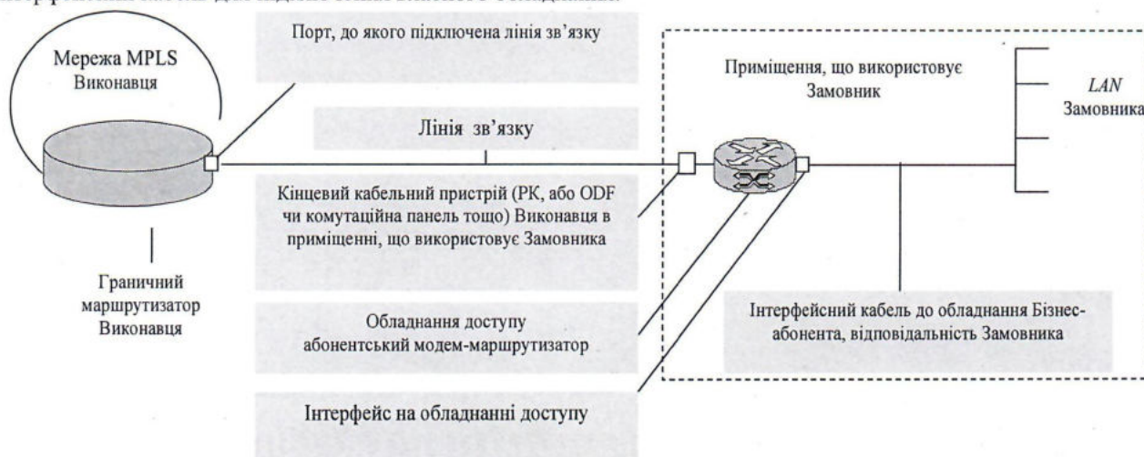
Рис. Конфігурація та схема надання Послуги ВПМ (Примітка: у разі інших умов підключення рисунок змінюється відповідно до домовленостей з Замовником)
